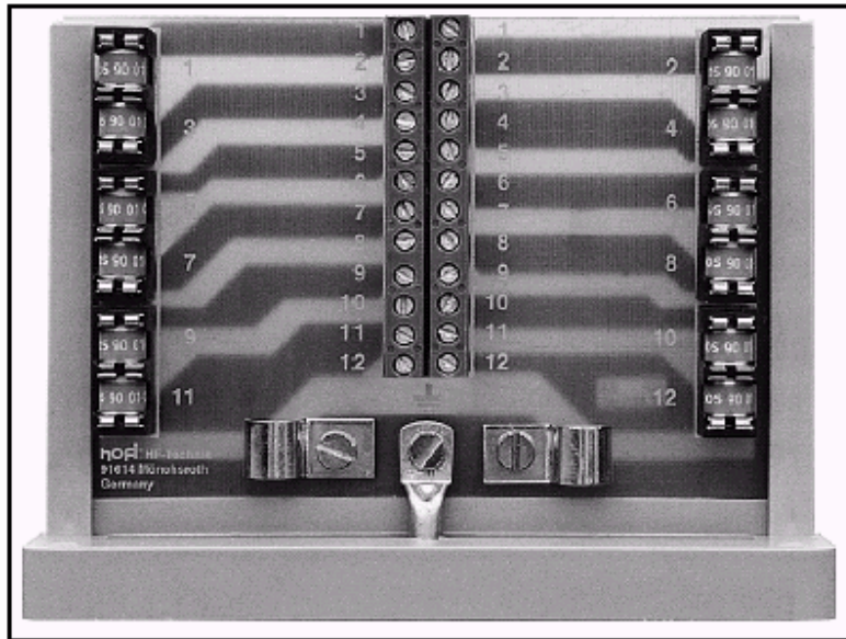
Bild 2:12-poliger Überspannungsableiter (hofl)
