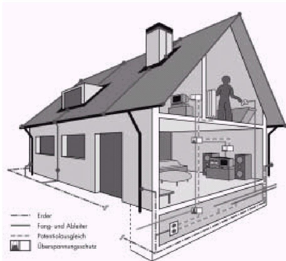
Bild 4: Blitzschutz-System:
